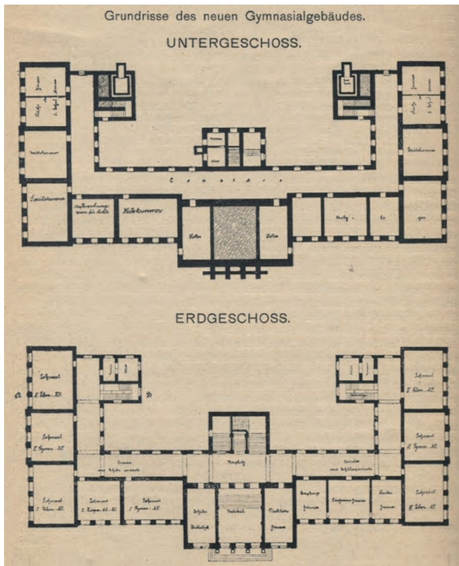
Grundrisse des neuen Gymnasialgebäudes: Untergeschoss und Erdgeschoss Quelle: Georg Fischer
